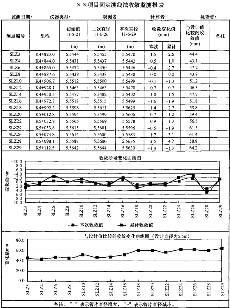
图 41 固定测线法收敛监测报表和变化曲线图
