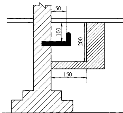
图 32 窨井式标志
