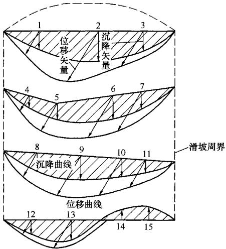
图 28 某斜坡监测点位移综合曲线图
